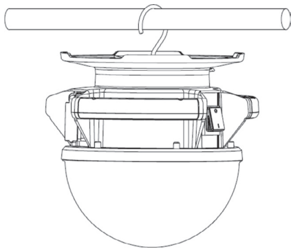
Ripustus
