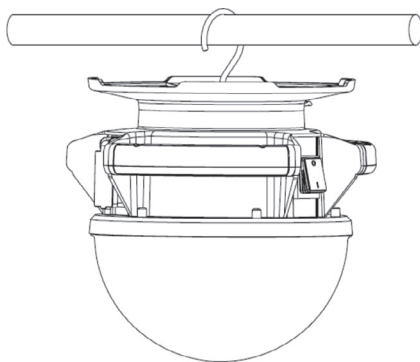
Upphängning
