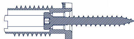
Föregående design med mindre kontaktyta och mindre kraftöverföring.
