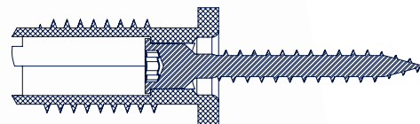
Nya designen med förbättrad kontaktyta för bättre kraftöverföring.
